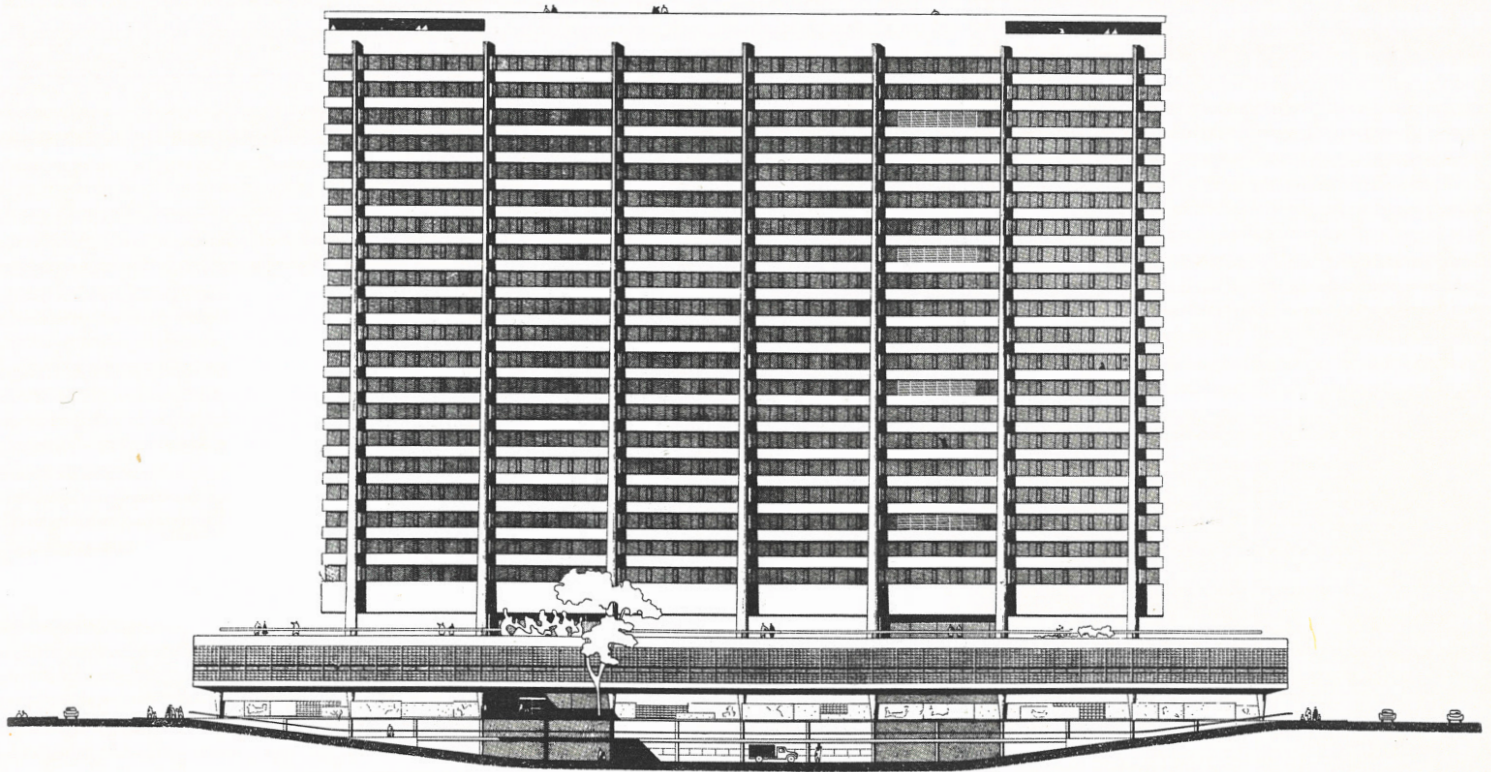
NOORD-OOSTGEVEL
