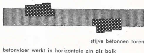
Figuur 2 Plattegrond willekeurige verdieping stijve betonnen toren
