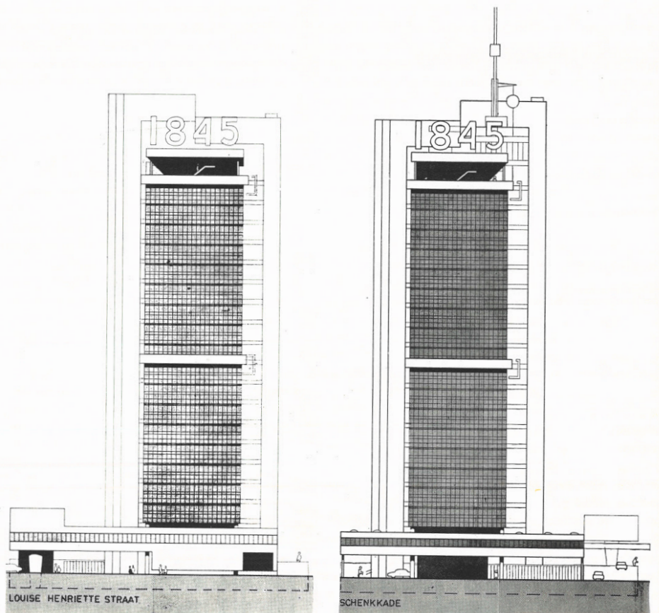
ZIJGEVELS
