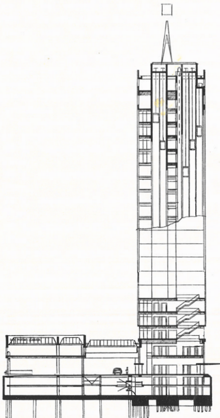
DWARSDOORSNEDE
