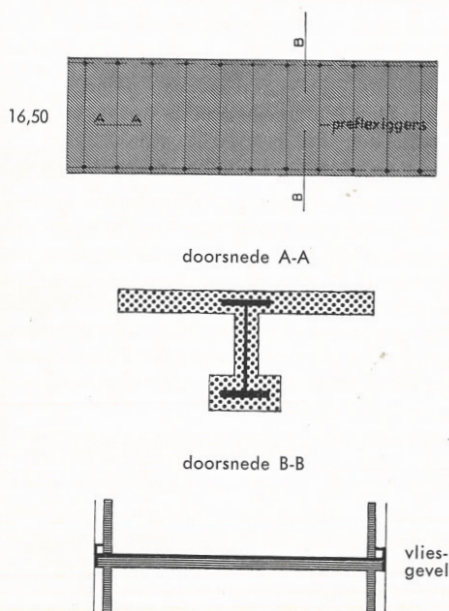
Figuur 1 Plattegrond schema vloerconstructie
