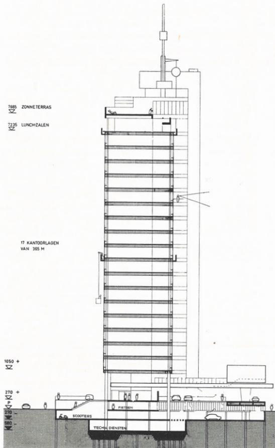
DWARSDOORSNEDE
